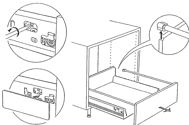
Etulevyn irroitus
